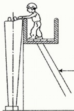
図4-1 架設施工時谷側足場
