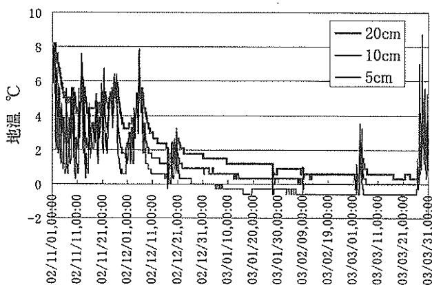
図5 対照区(cont1) 深度別地温変化
