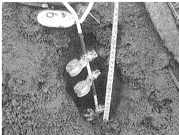
写真8 地温計埋設状況
