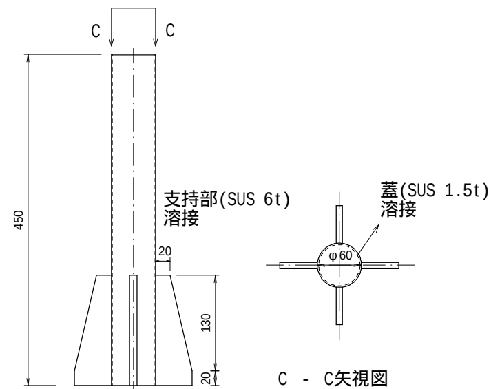
パイプスタンプ図
