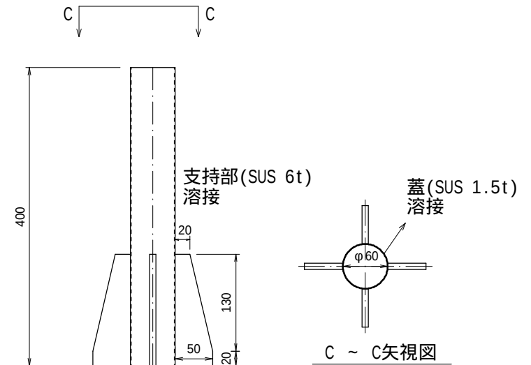
パイプステーション図
