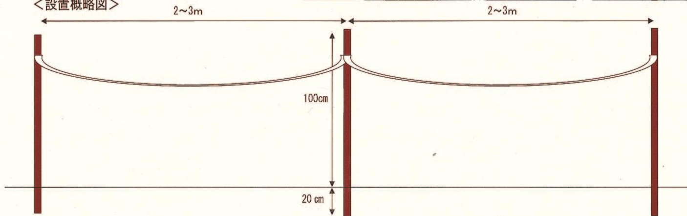
<設置概略図>
