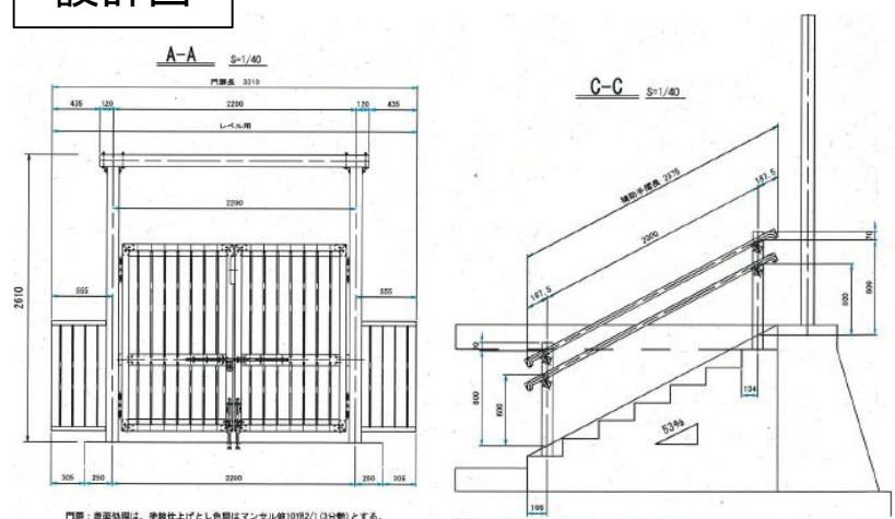
設計図
