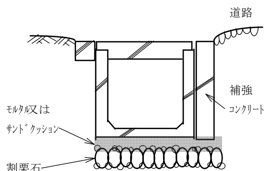
第6図 (標準図)
