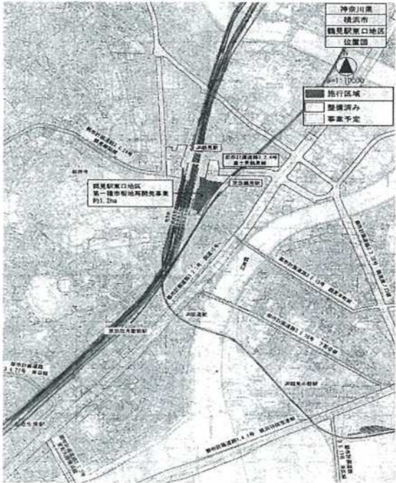
位置図
