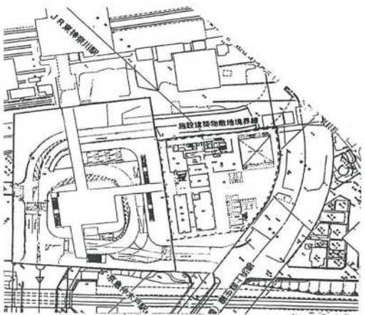
配置図
