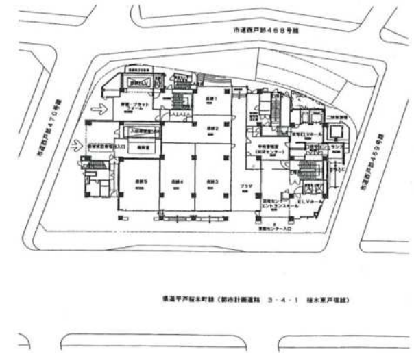
配置図
