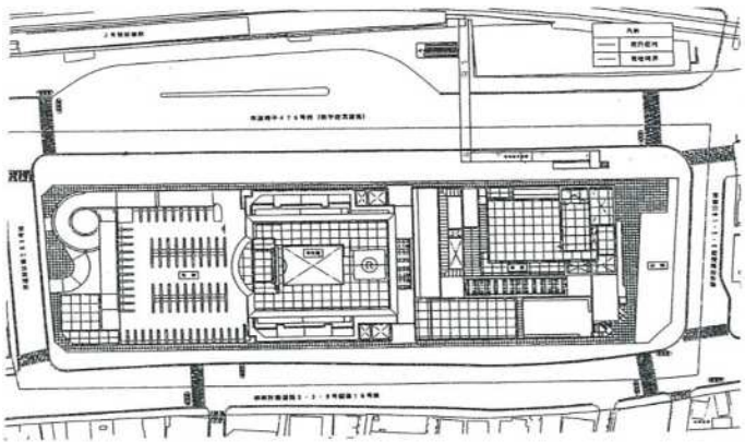
配置図
