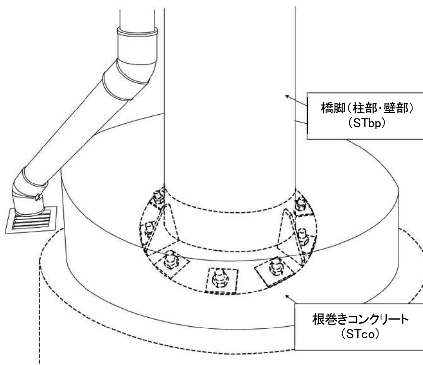
付図－１． １． １ 部材の名称（その４）
