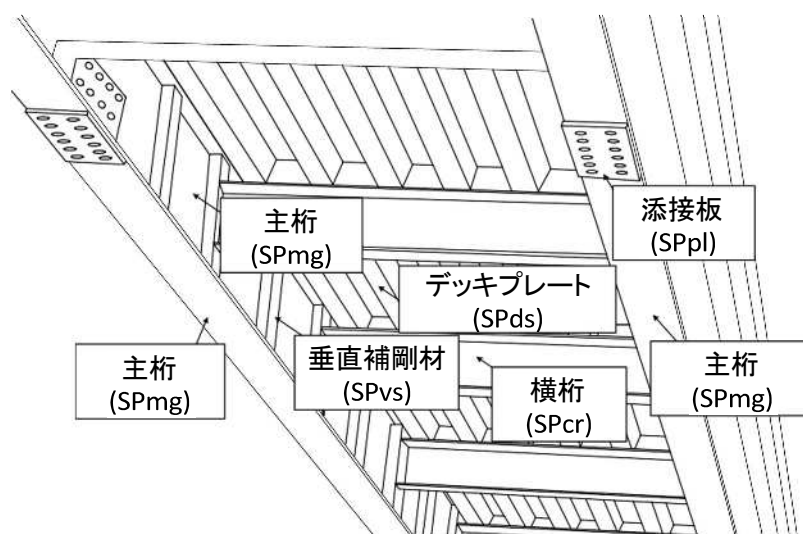
デッキプレート形式②
