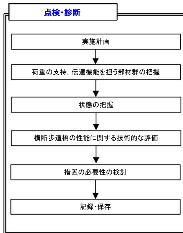
図－１．１ 点検・診断に関連するフロー
