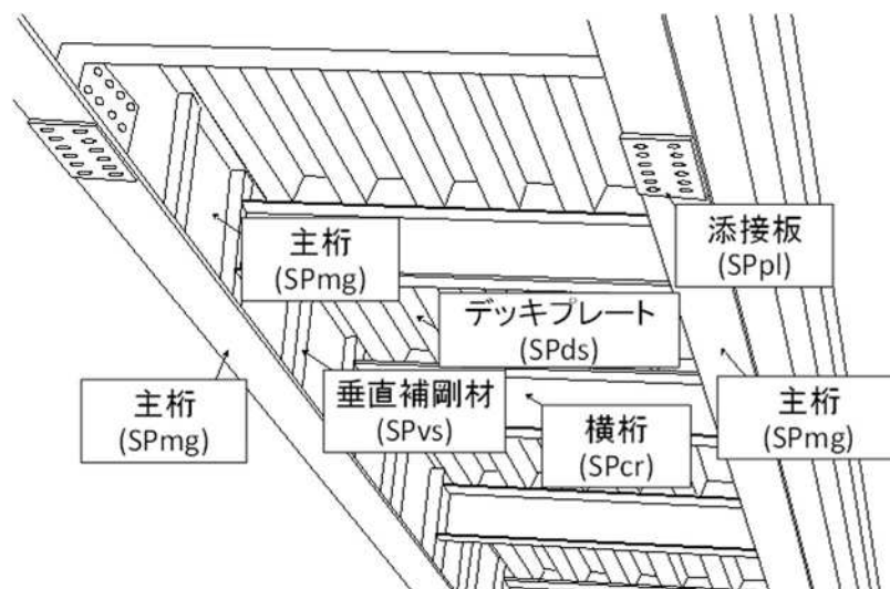
付図－１．１．１ 部材の名称（その１）
