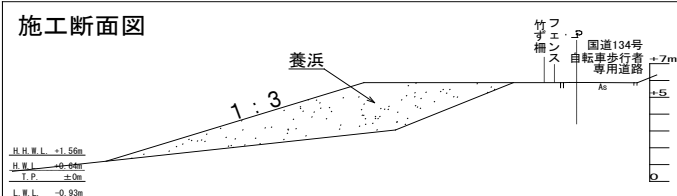
将来断面図
