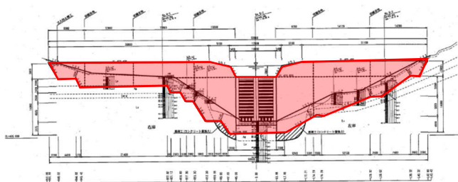
【堰堤工正面図】 （計画-9 堰堤）
