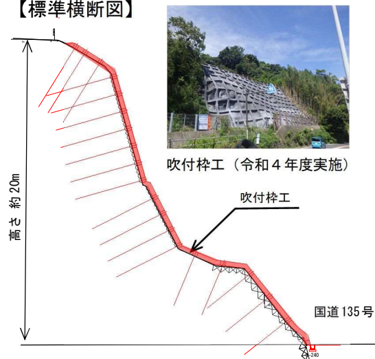
【標準横断面図】
