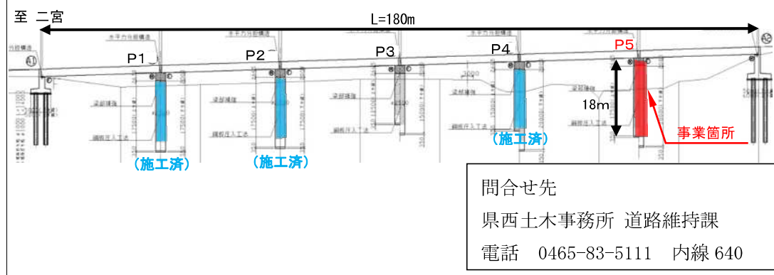
【立面図】
