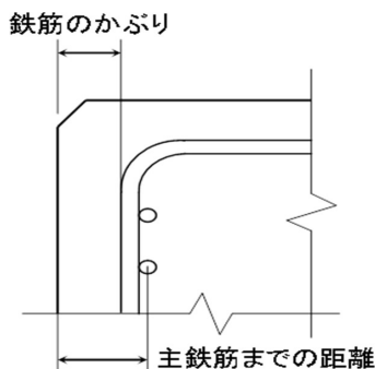
図1-3-1 鉄筋のかぶり
