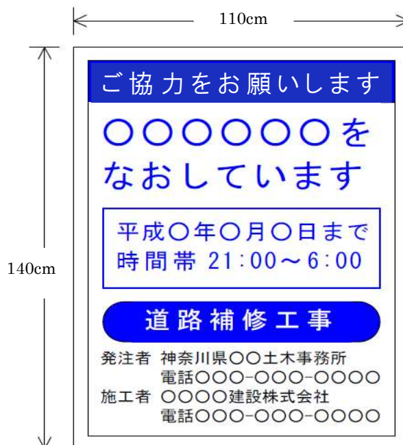
図1-1-2 工事中標示板の標準図
