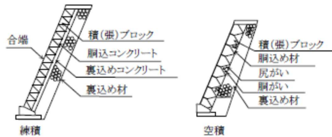
図 3-2-5 コンクリートブロック工
