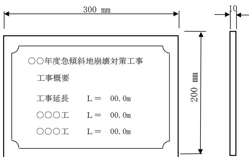
図 6-4-1 工事概要板
