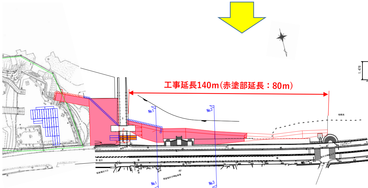
図2 令和6年度の養浜位置及び断面
