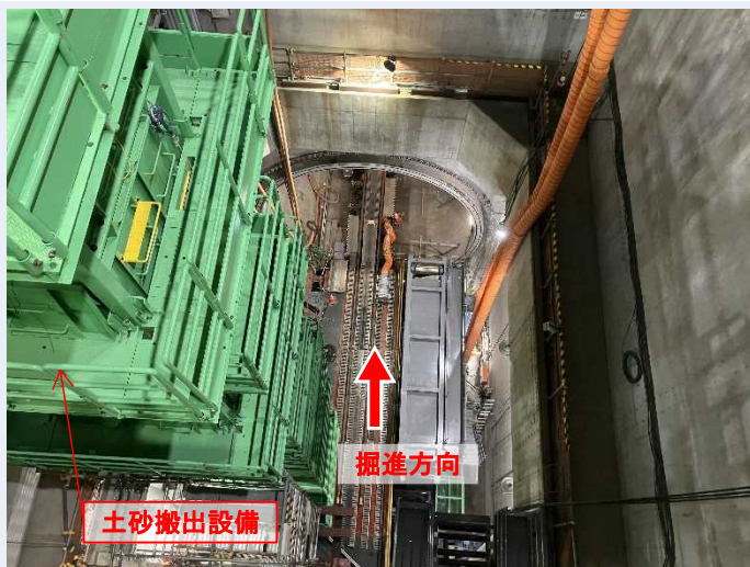
発進立坑内
