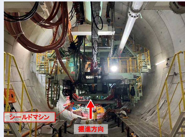
トンネル坑内(100m地点)
