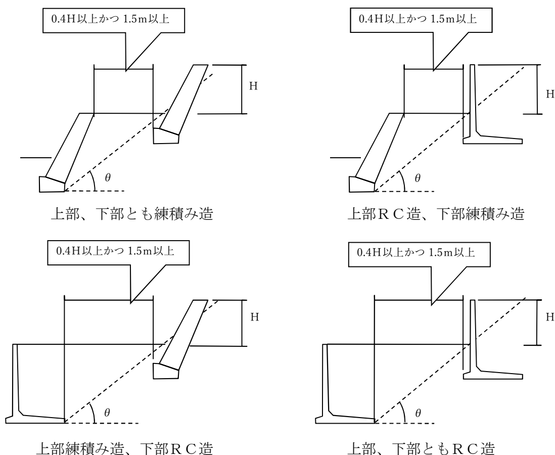
【図Ⅲ. 2-6 多段擁壁の考え方(上段擁壁がθの範囲外のものを多段擁壁とする)】
