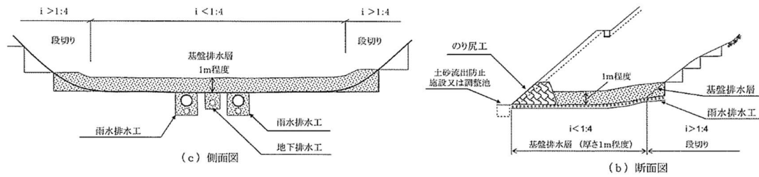
【図Ⅲ. 1－3 基底排水層の設置例】
