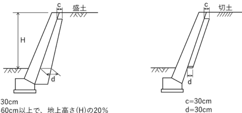
【図Ⅱ. 2-17 裏込め材の配置】
