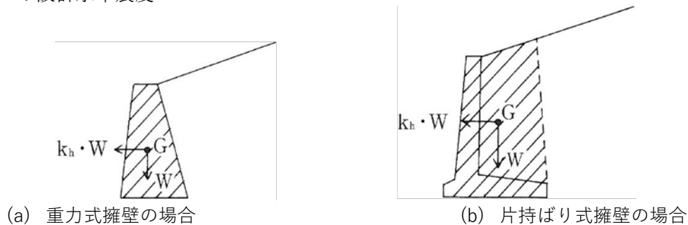
【図Ⅱ. 3-8 地震時慣性力の考え方】
