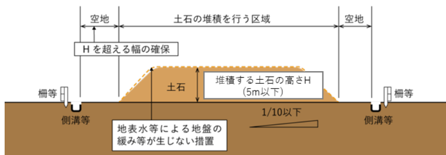
【図 II. 7-2 堆積する土地の基準（高さ 5m 以下）】
