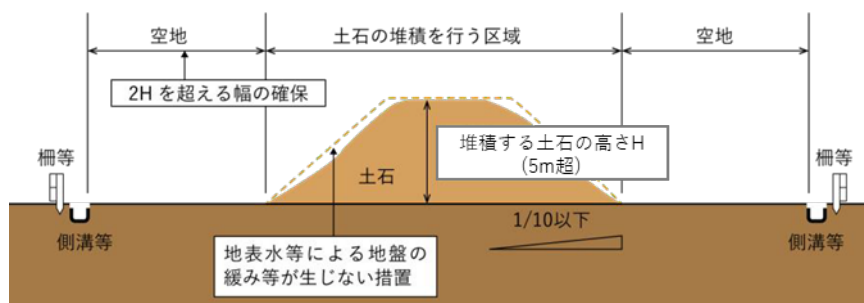
【図 II. 7-3 堆積する土地の基準（高さ 5m 超）】
