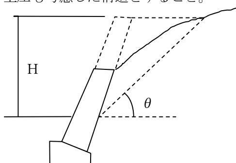
【図Ⅱ. 2-5 上部に斜面がある場合の擁壁の構造（練積み造の場合）】
