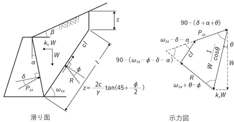
【図Ⅱ. 3-7 裏込め土が粘着力を有する場合の地震時主働土圧】
