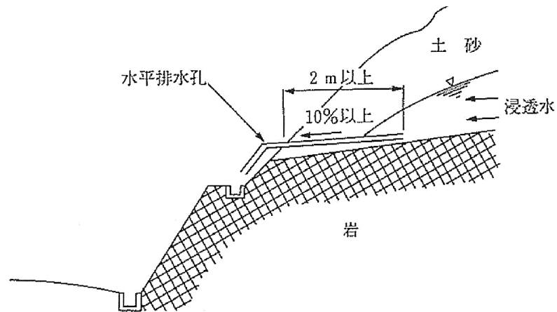
【図Ⅱ. 6-22 水平排水孔の例】 『盛土等防災マニュアルの解説 盛土等防災研究会』
