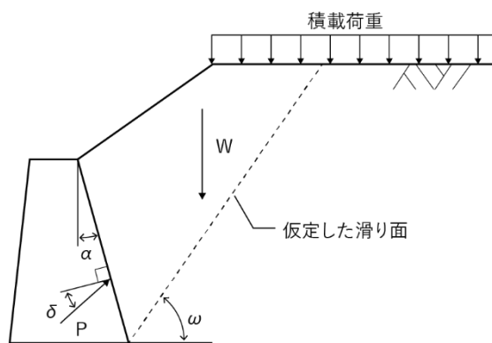
【図Ⅱ. 3-5 試行くさび法】
