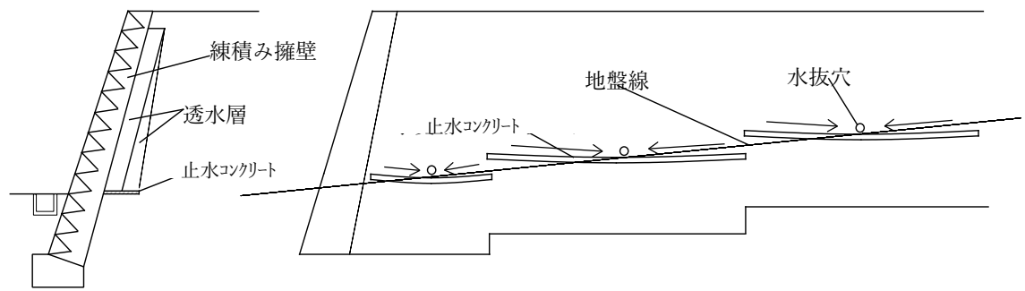
【図Ⅱ. 2-12 止水コンクリート】
