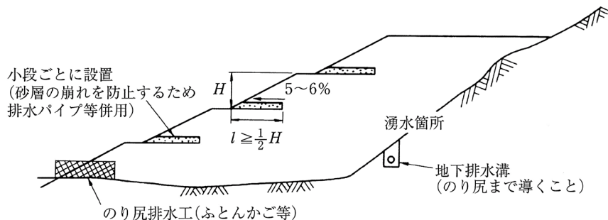
【図Ⅱ. 6-11 水平排水層の例】
