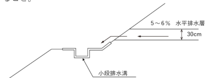
【図Ⅱ. 6-10 水平排水層端末部】
