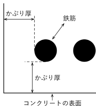
【図Ⅱ. 2-14 鉄筋のかぶり厚さ】
