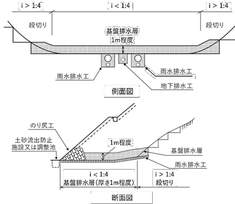
【図Ⅱ. 6-9 基盤排水層の設置例】
