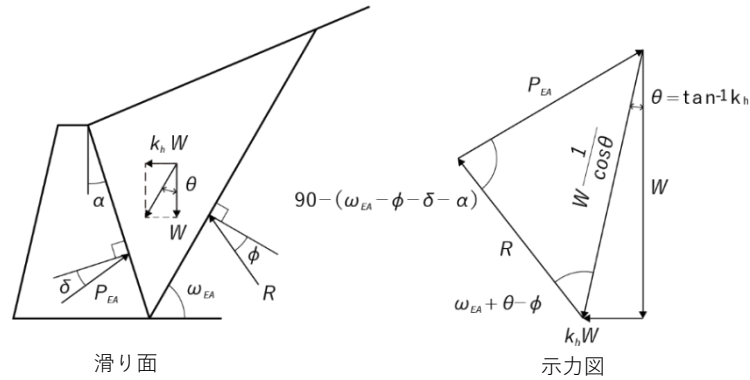
【図Ⅱ. 3-6 地震時主働土圧の考え方】
