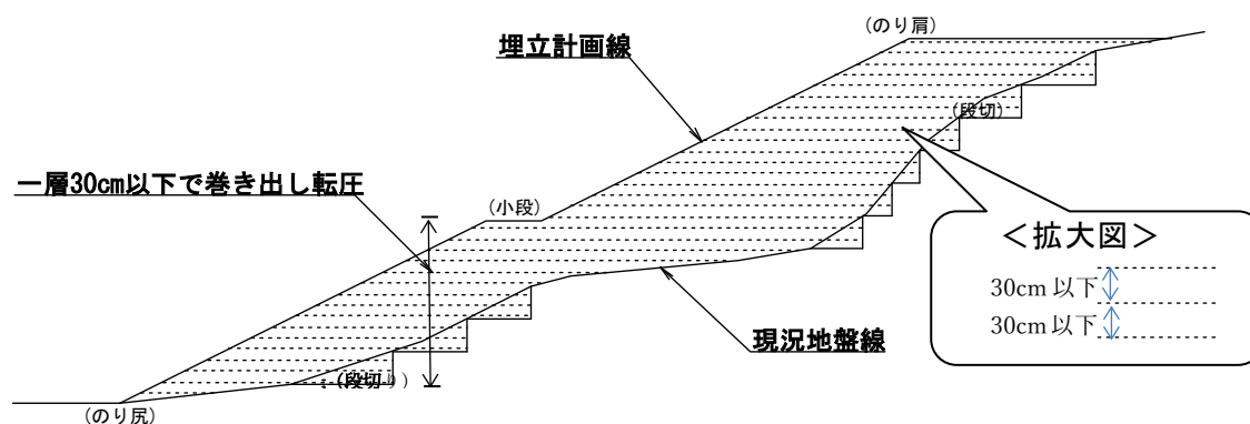
【図Ⅱ. 1－1 土砂の巻出し及び転圧方法（標準図）】
