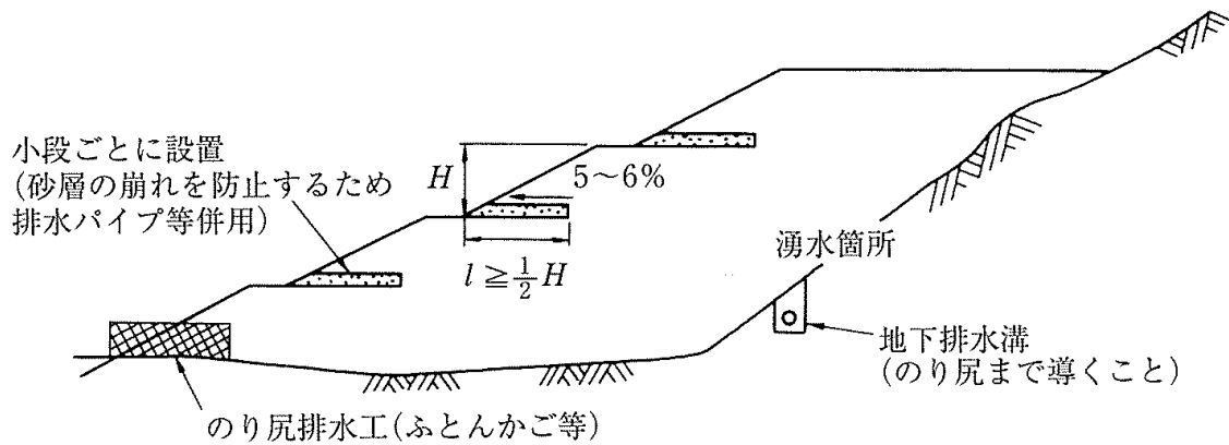
【図Ⅱ. 1－4 水平排水層の設置例】
