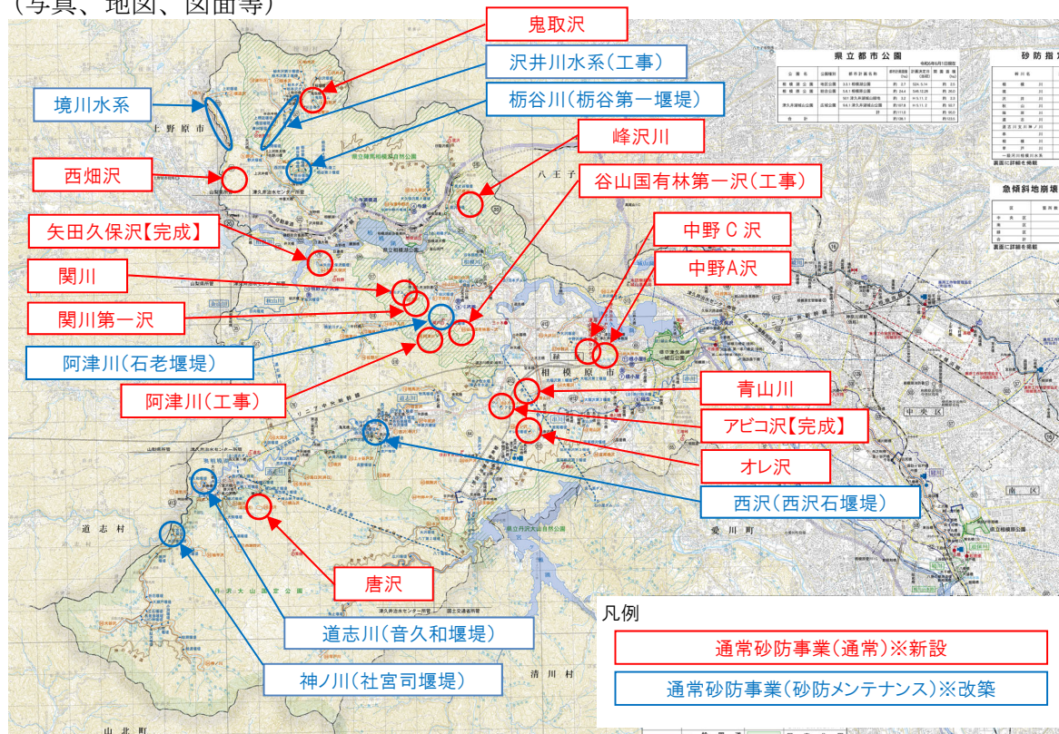
【矢田久保沢（令和3年度完成）】
